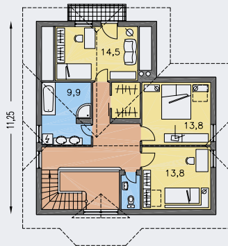
POSCHODÍ [plocha 74.4 m 2 ]
