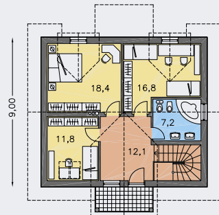
poschodí [plocha 71.4 m 2 ]
