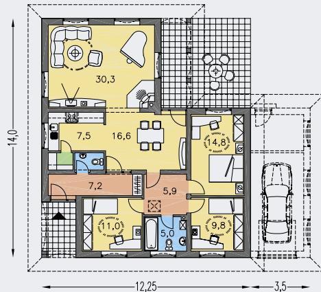
PŘÍZEMÍ [plocha 111.3 m 2 ]
