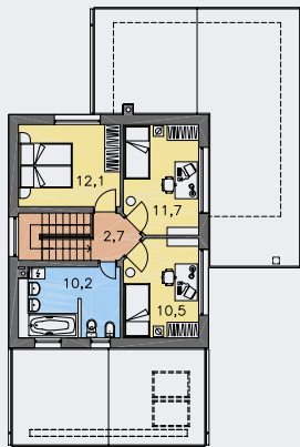
POSCHODÍ [plocha 47.3 m 2 ]
