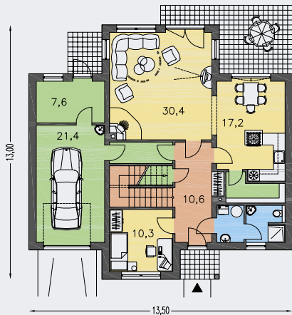
PŘÍZEMÍ [plocha 121.0 m 2 ]
