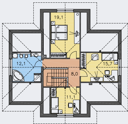
POSCHODÍ [plocha 66.0 m 2 ]
