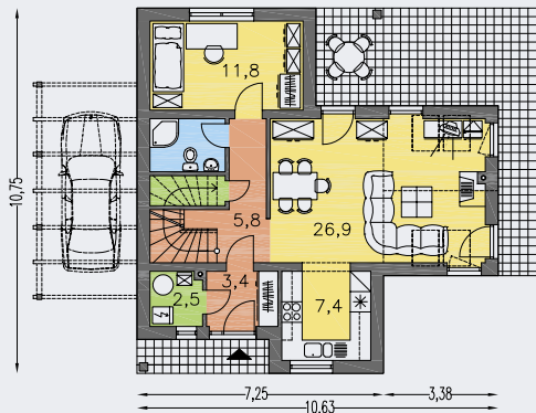
PŘÍZEMÍ [plocha 67.6 m 2 ]
