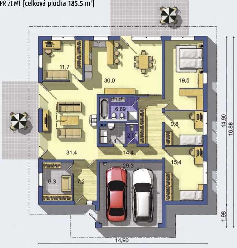
PŘÍZEMÍ [celková plocha 185.5 m 2 ]
