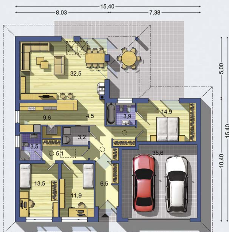
PŘÍZEMÍ [celková plocha 154.6 m 2 ]
