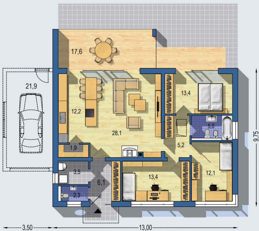
PRÍZEMÍ [celková plocha 103.3 m 2 ]
